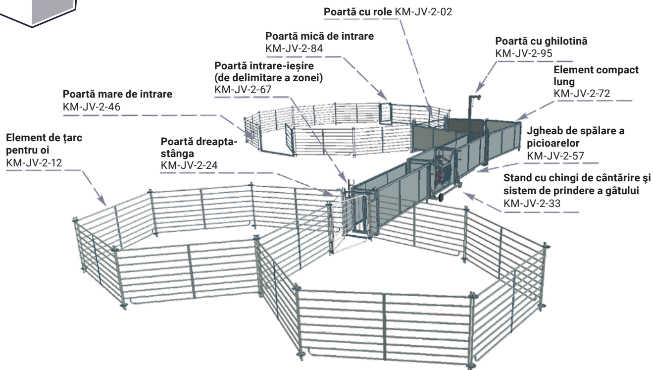
Sistem de sortare ovine 0001 | KM-JV-2-0001
