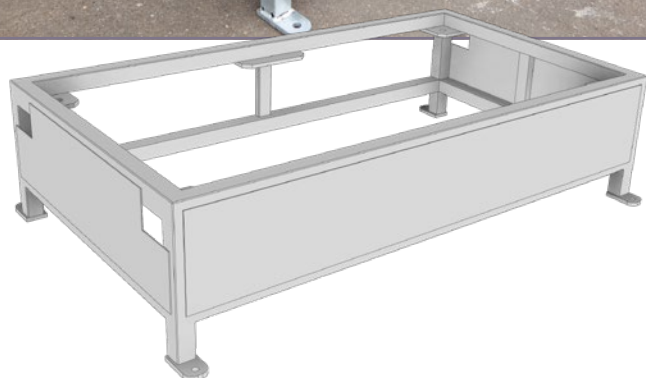
Suport pentru adăpătoare dublă Erinox KM-MI-ERXD110-HOLD
