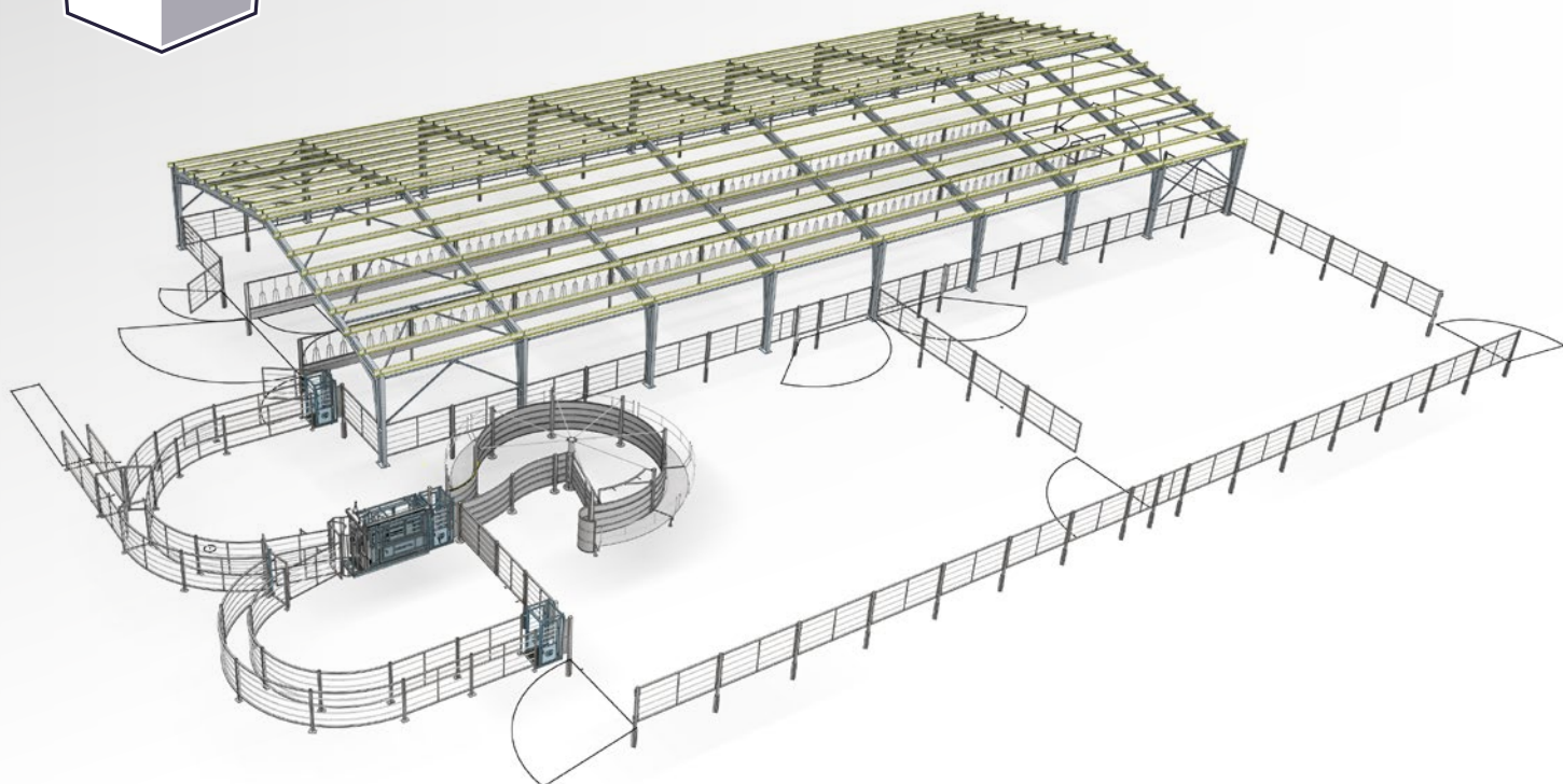
Clădire hambar deschis cu sistem de selecție 20 m x 48 m x 4 m | Locul construcției: Pusztaföldvár
