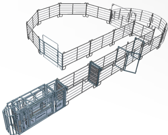
Sistem complet de sortare 8001 | KM-MV-4-8001
