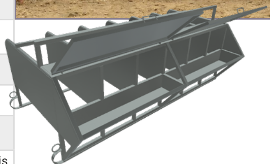
lesle pentru baloți rotunzi cu 12 locuri de hrănire, întărită, acoperită complet cu foi de metal | KM-MB-BOX06-H
