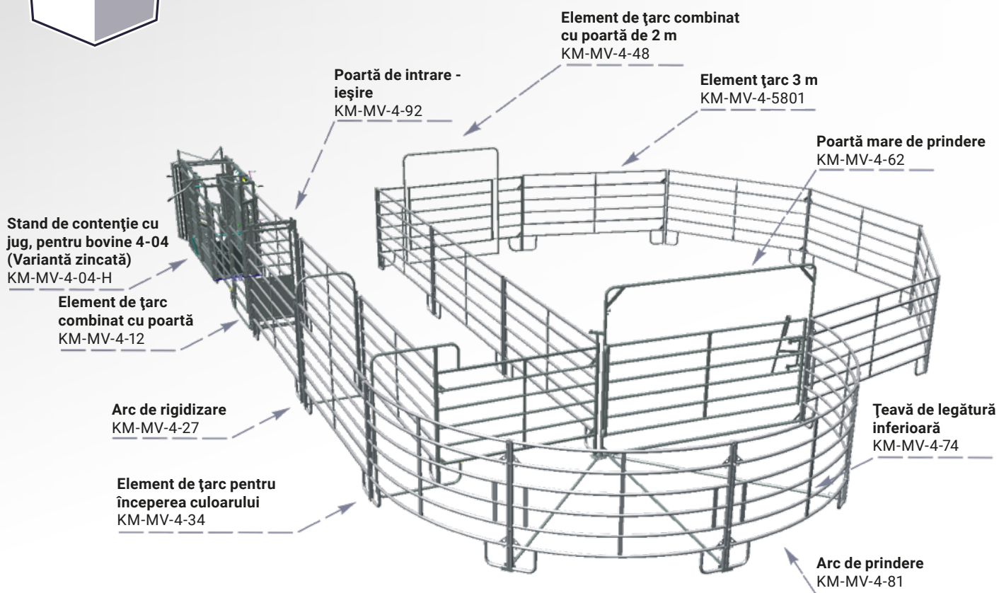
Sistem complet de sortare 8001 | KM-MV-4-8001
