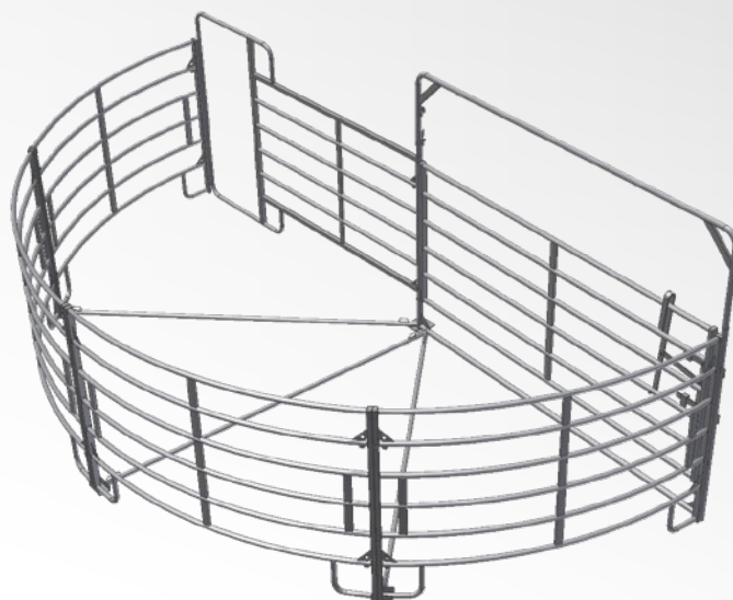
Set de dirijare cu 4 panouri curbate | KM-MV-4-8104
