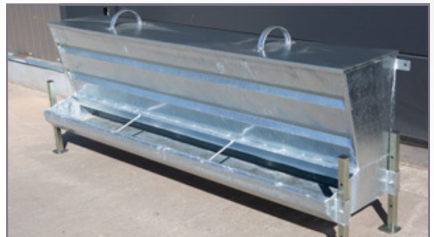
Hranitor pentru oi cu rezervor (L=2 m, cu acoperis) KM-JE-3-32OSWR
