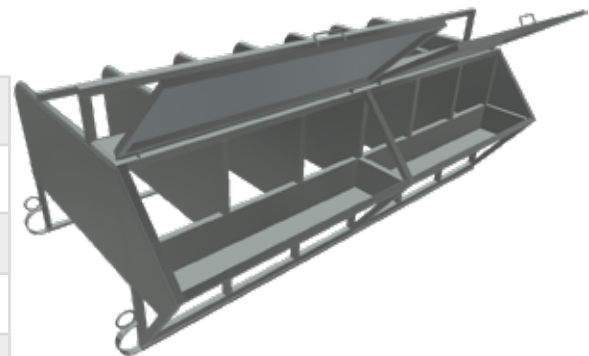
Cresa de vitei cu boxe pentru 6 vitei (galvanizat la cald) | KM-MB-BOX06-H
